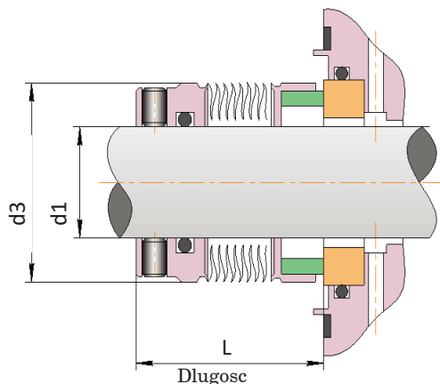
Mechaniczne uszczelnienie końcowe R-680 (676 / 670 / 680)
